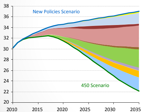
Global utslepp av CO 2 Samanlikning av to IEA scenario
